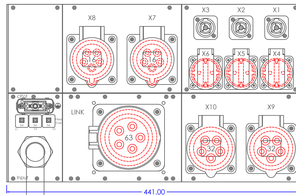
Ansicht Rückseite
