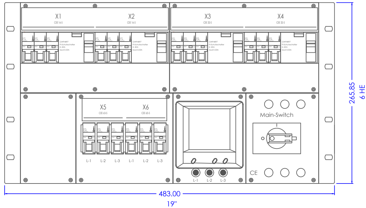
Ansicht Frontseite
