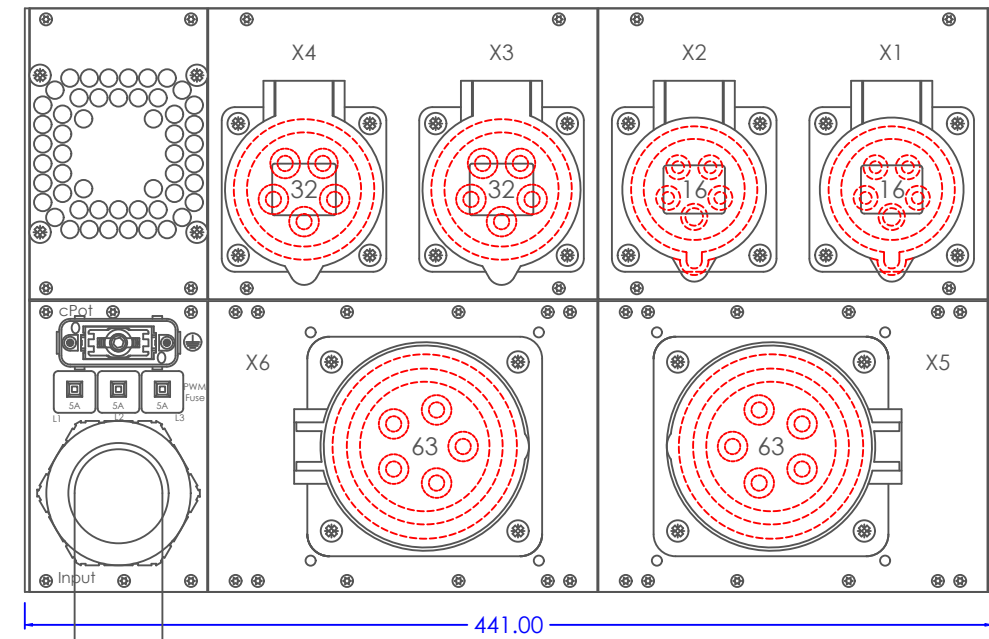
Ansicht Rückseite
