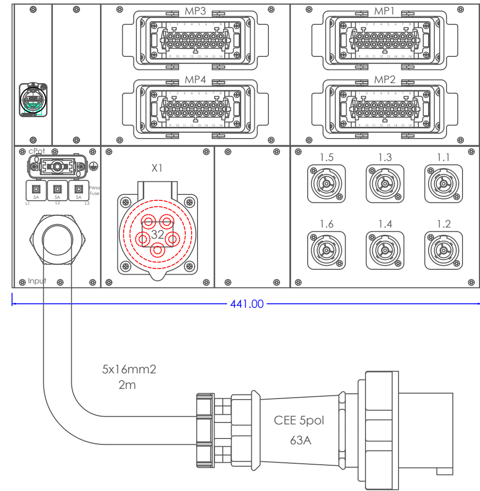
Ansicht Rückseite
